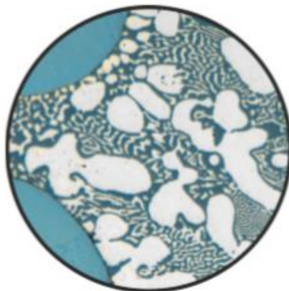
Mo-Cu-P Pseudolegierung
